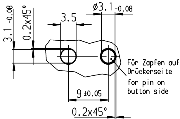
Empfohlenes Lochbild recommended hole pattern
