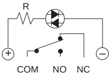
SPDT
